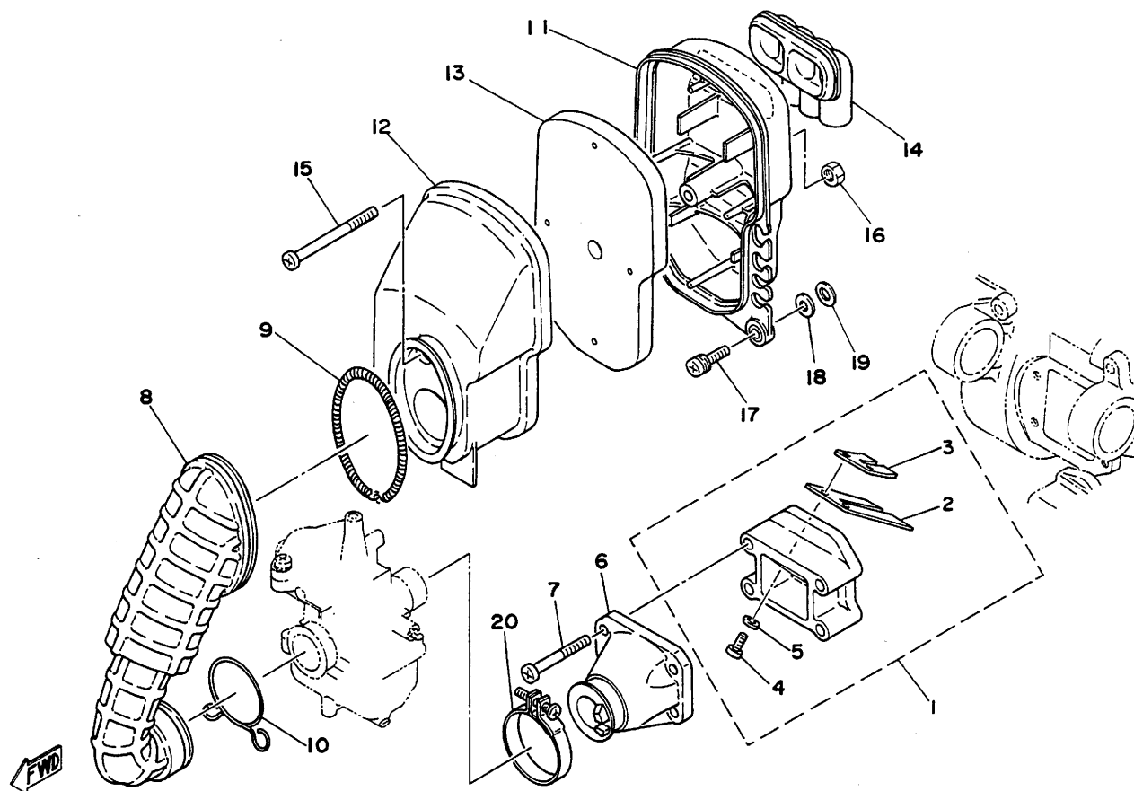
第6図 インテーク
