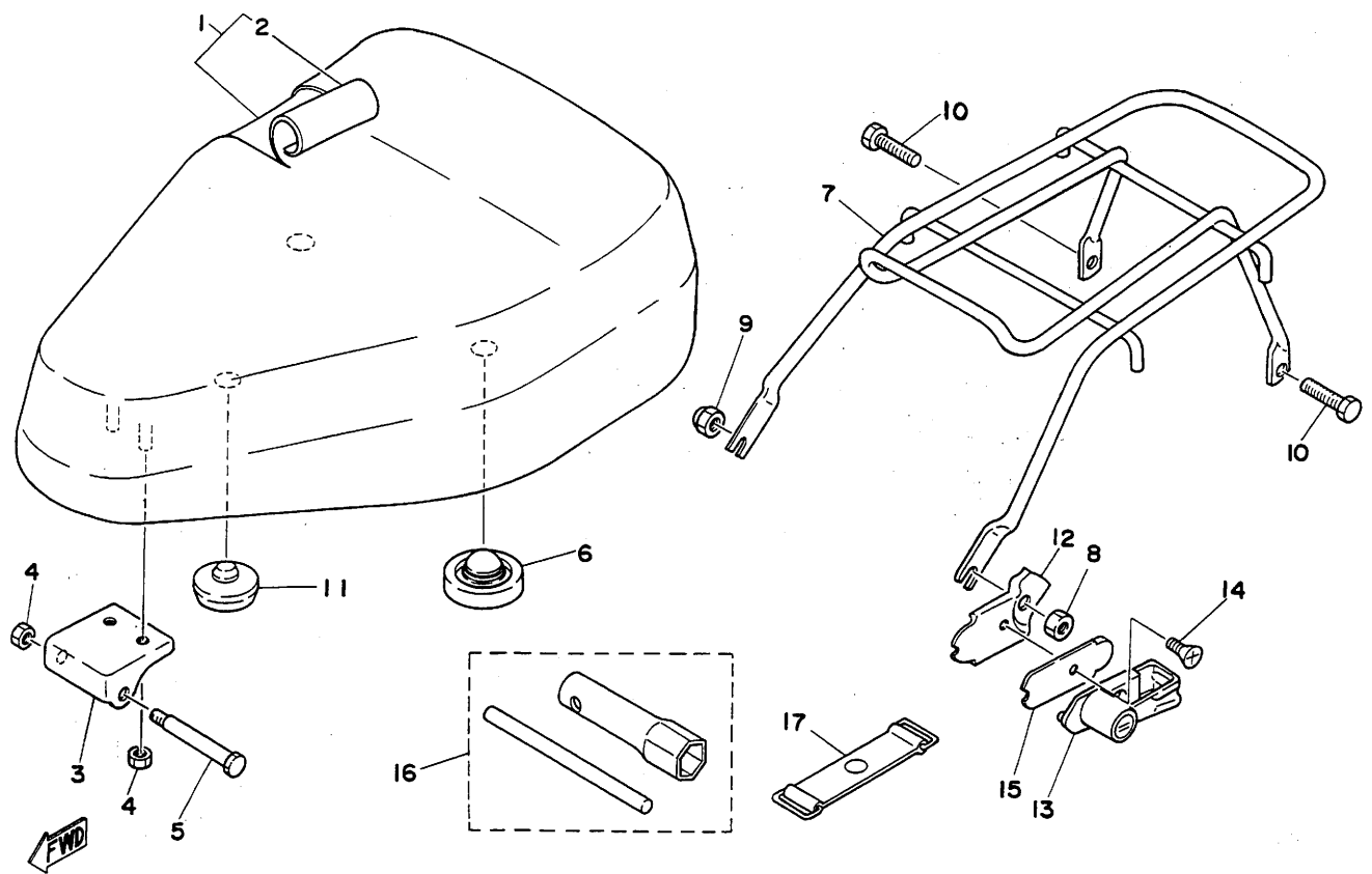
第22図 シート・ツール
