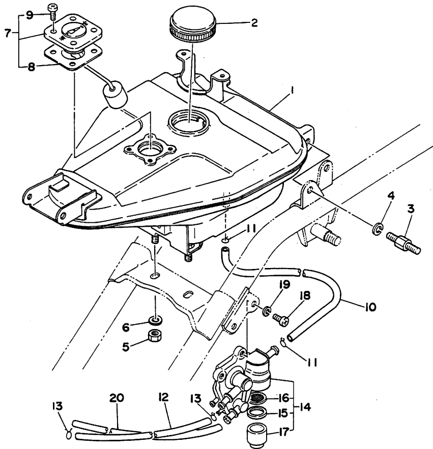
第21図 フュエルタンク
