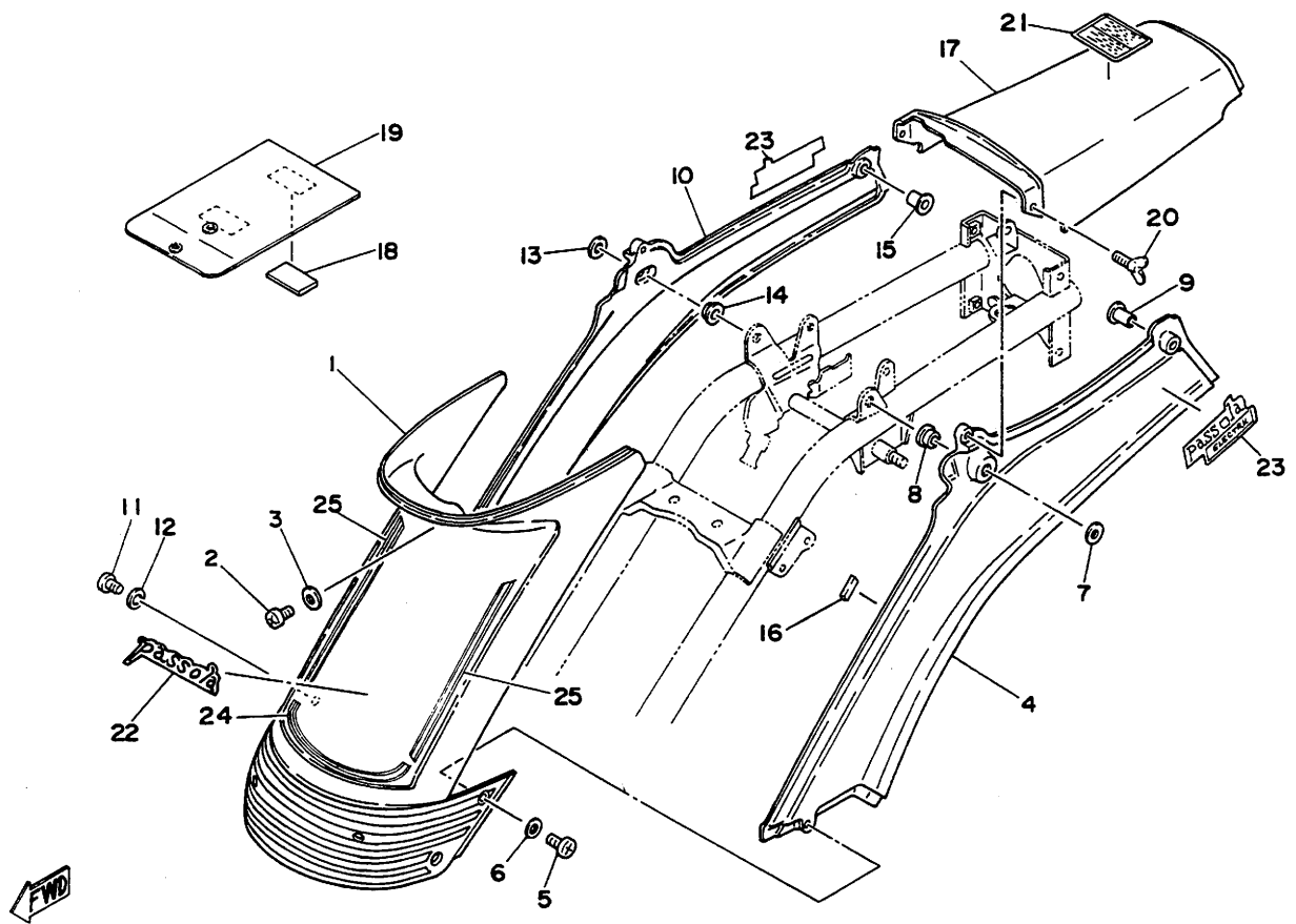
第16図 サイドカバー
