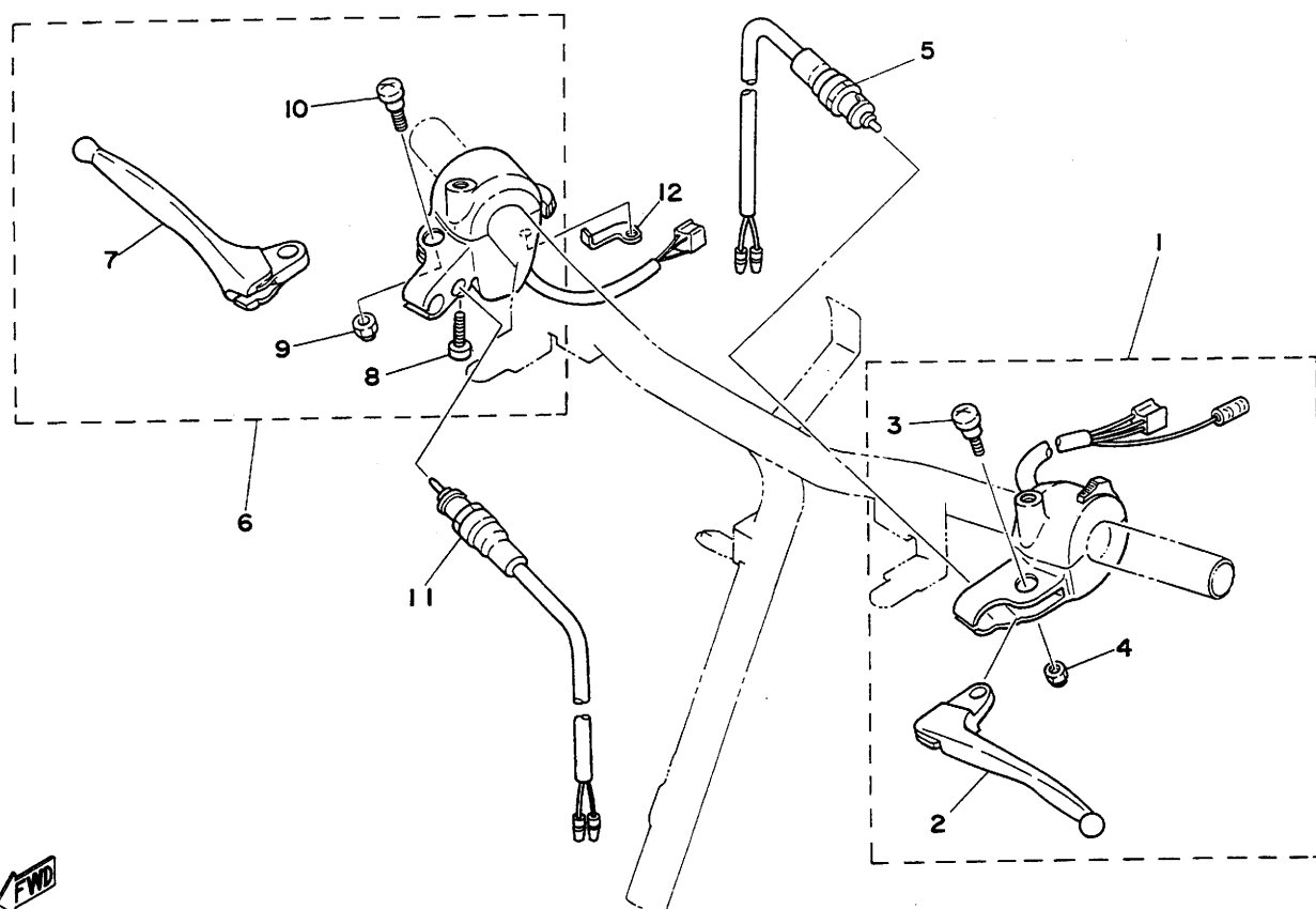
第34図 ハンドルスイッチ・レバー
