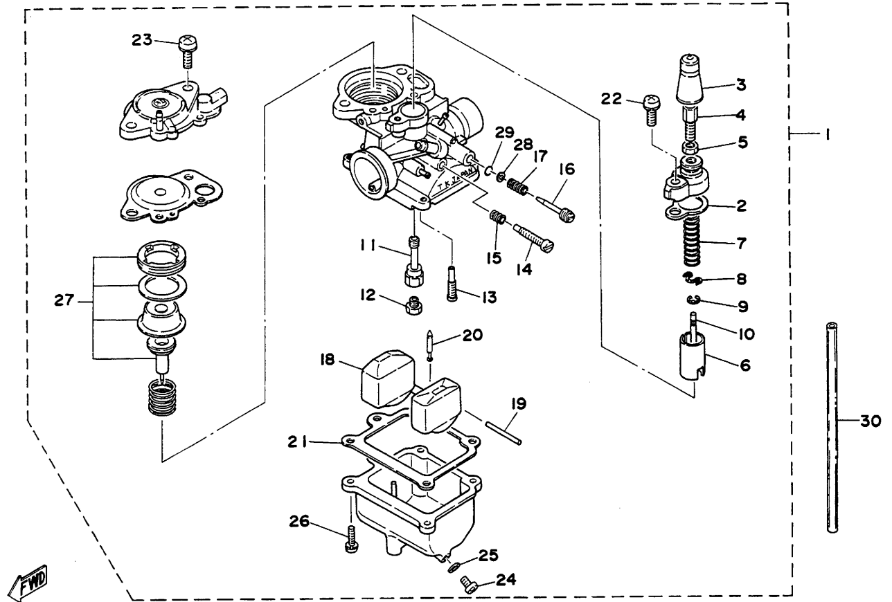
第7図 キャブレタ
