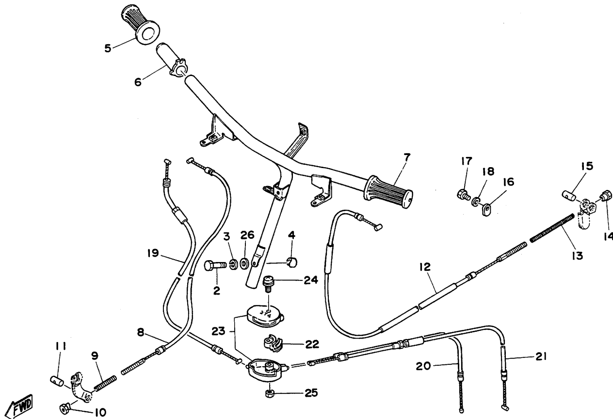
第25図 ステアリングハンドル・ケーブル
