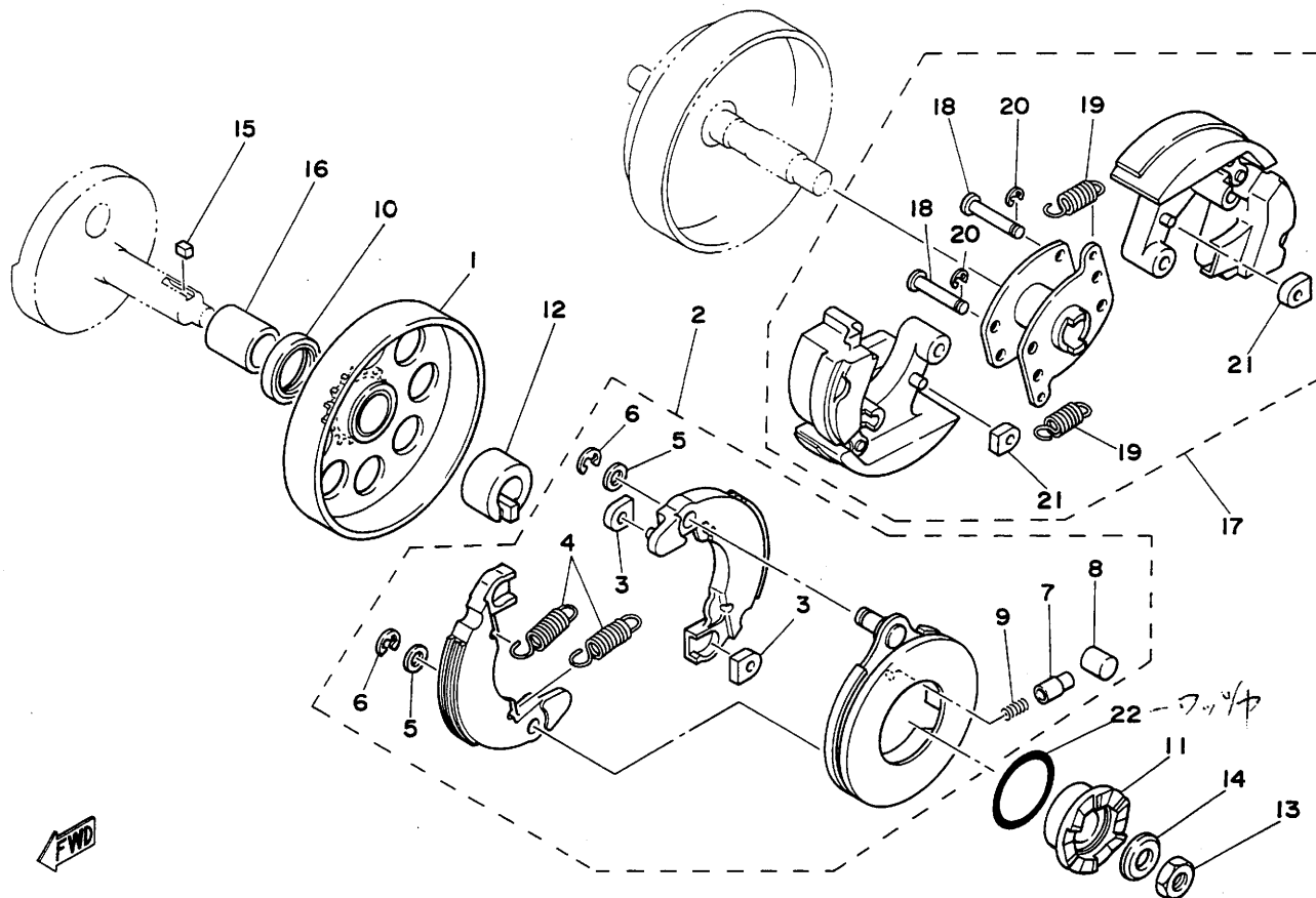
第12図 クラッチ
