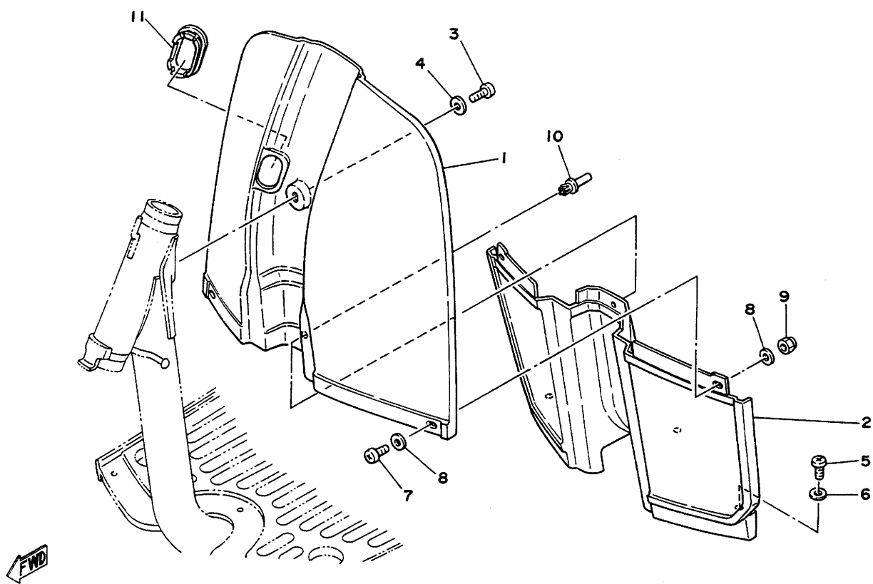
第28図 レッグシールド
