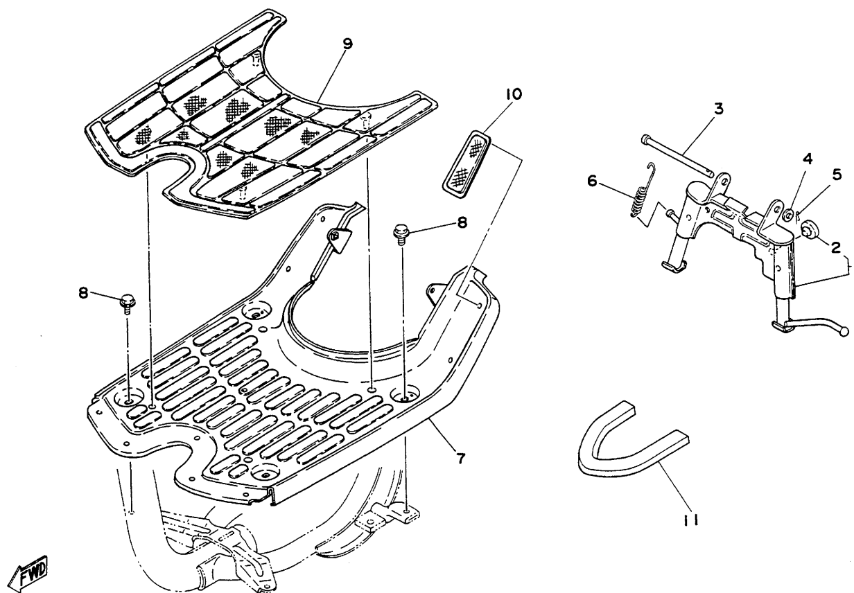
第27図 スタンド・フートレスト
