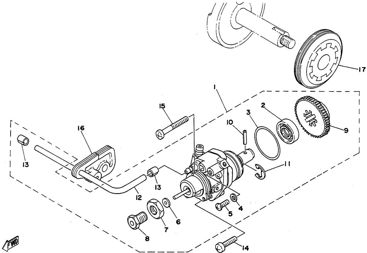
第5図 オイルポンプ
