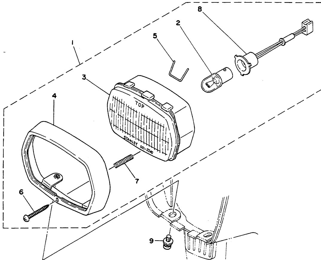
第31図 ヘッドライト
