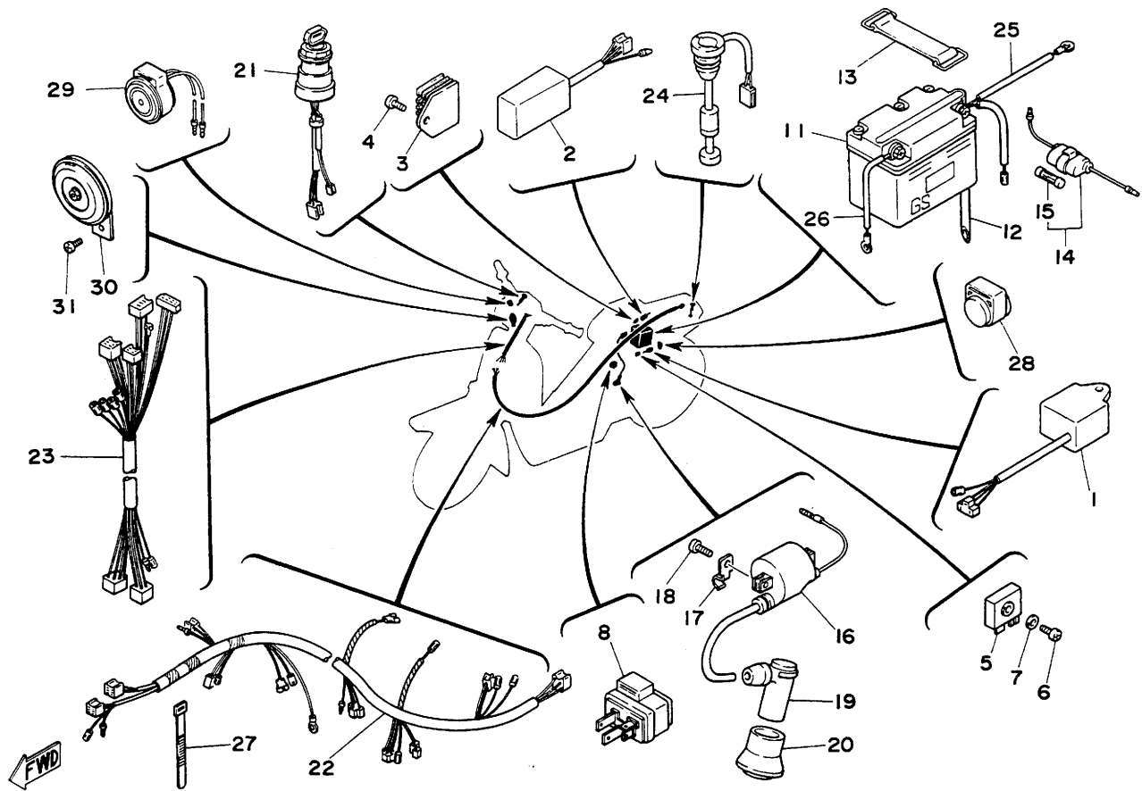
第33図 エレクトリカル 1
