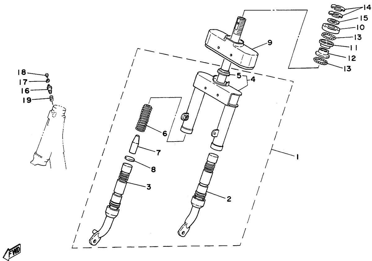
第19図 フロントフォーク
